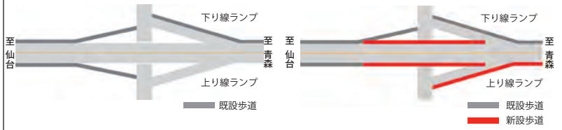
【現況図】
