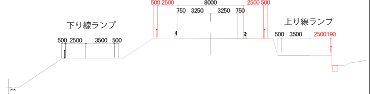
【計画横断面】
